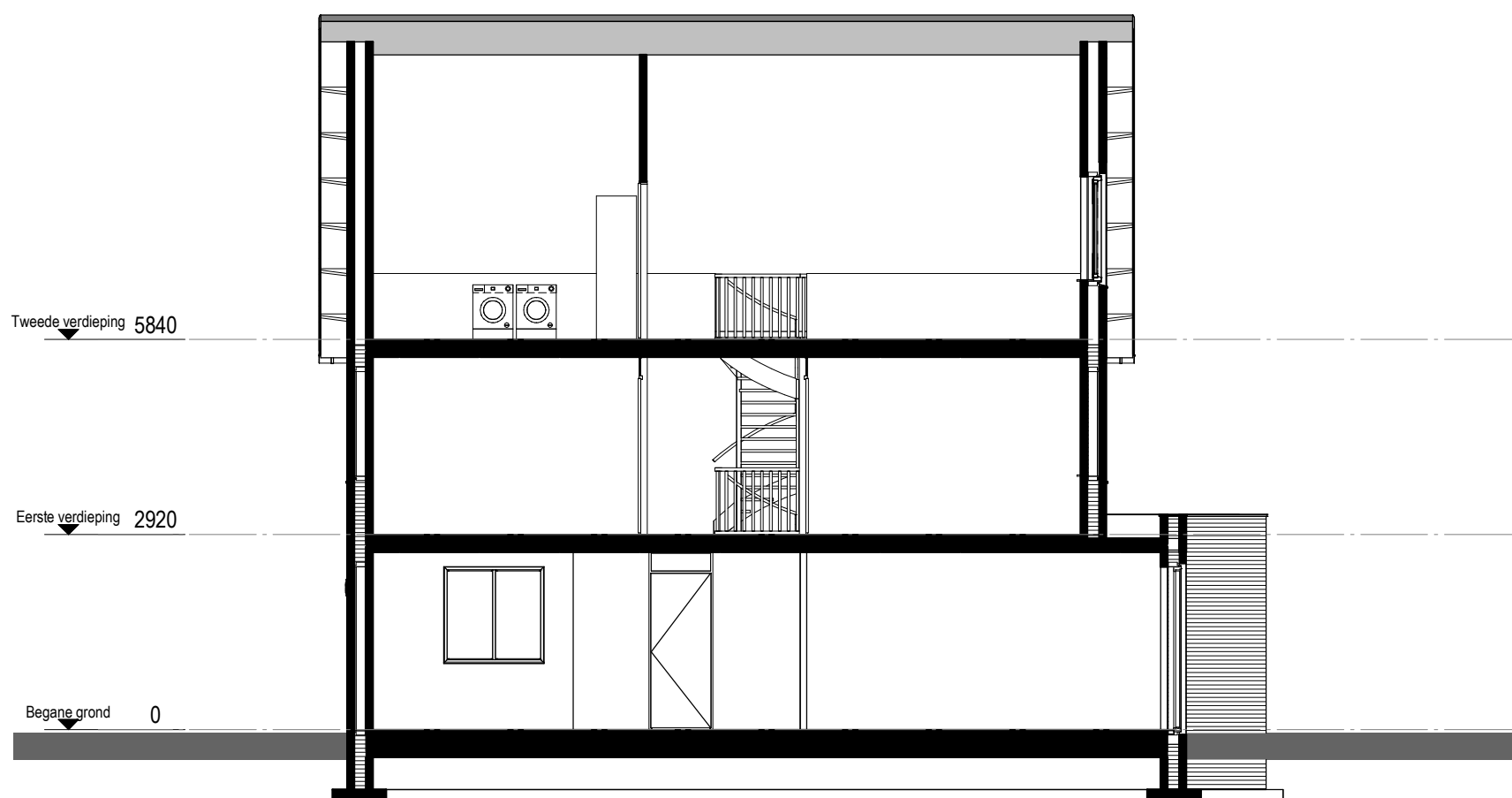
Doorsnede A
