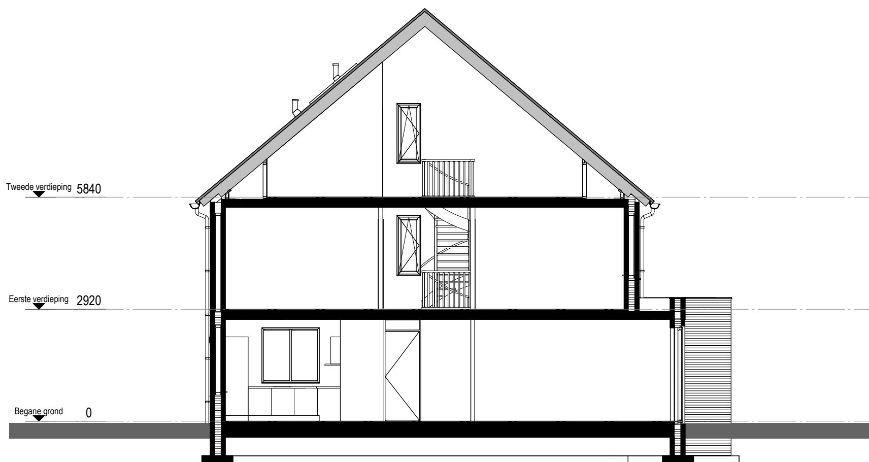
Doorsnede A
