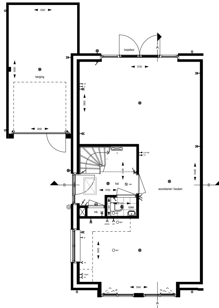
begane grond
