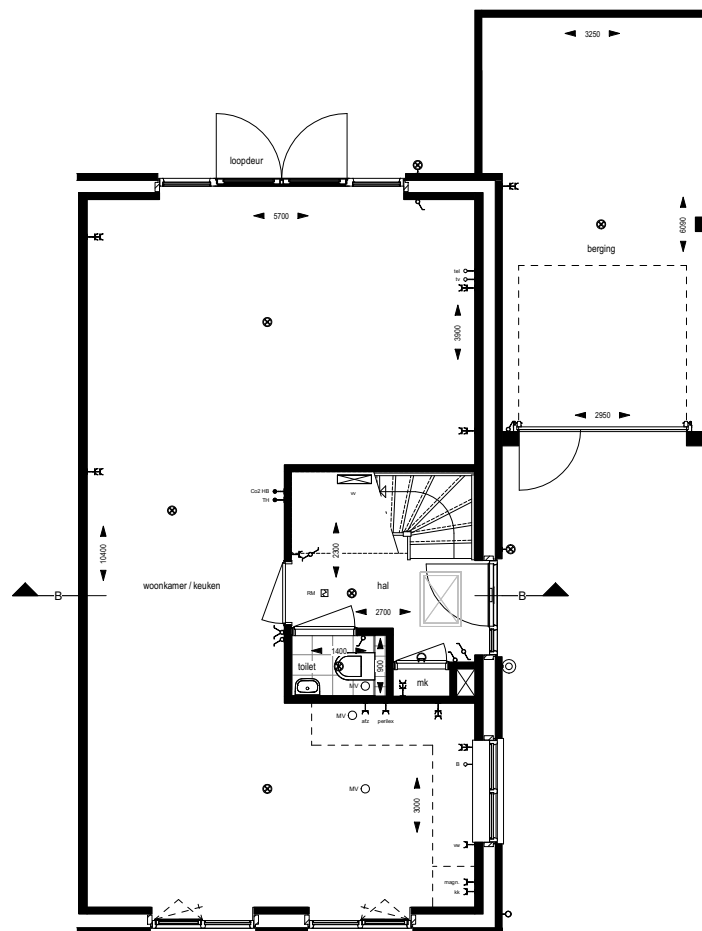
begane grond
