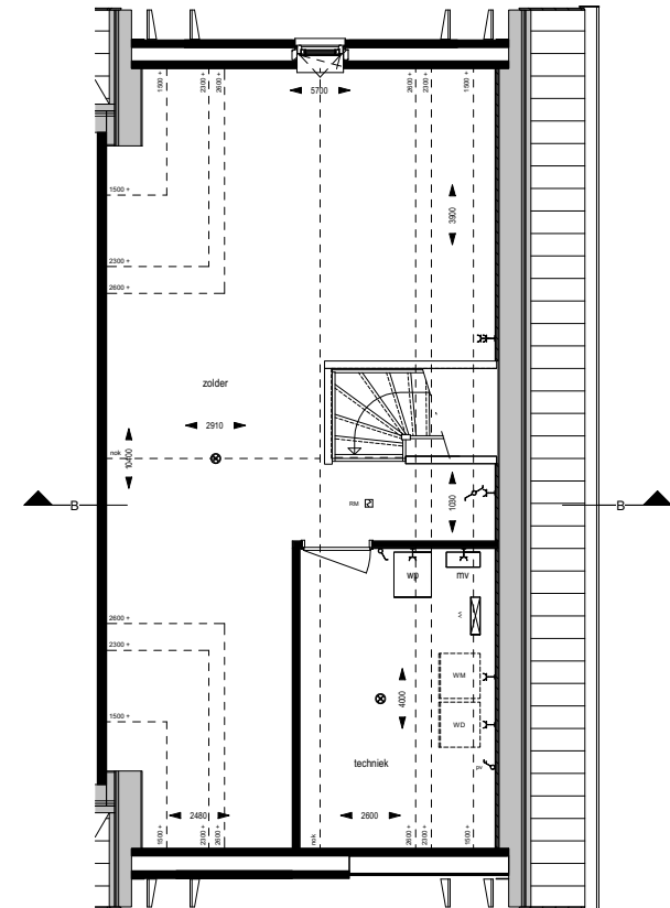
2 e verdieping
