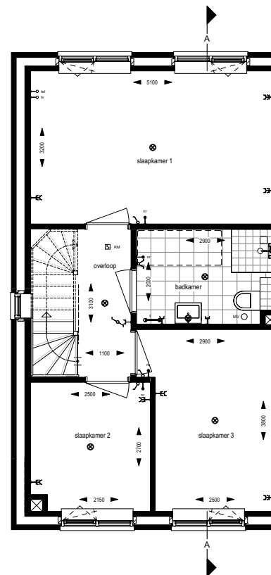
1 e verdieping
