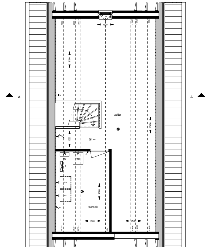
2 e verdieping
