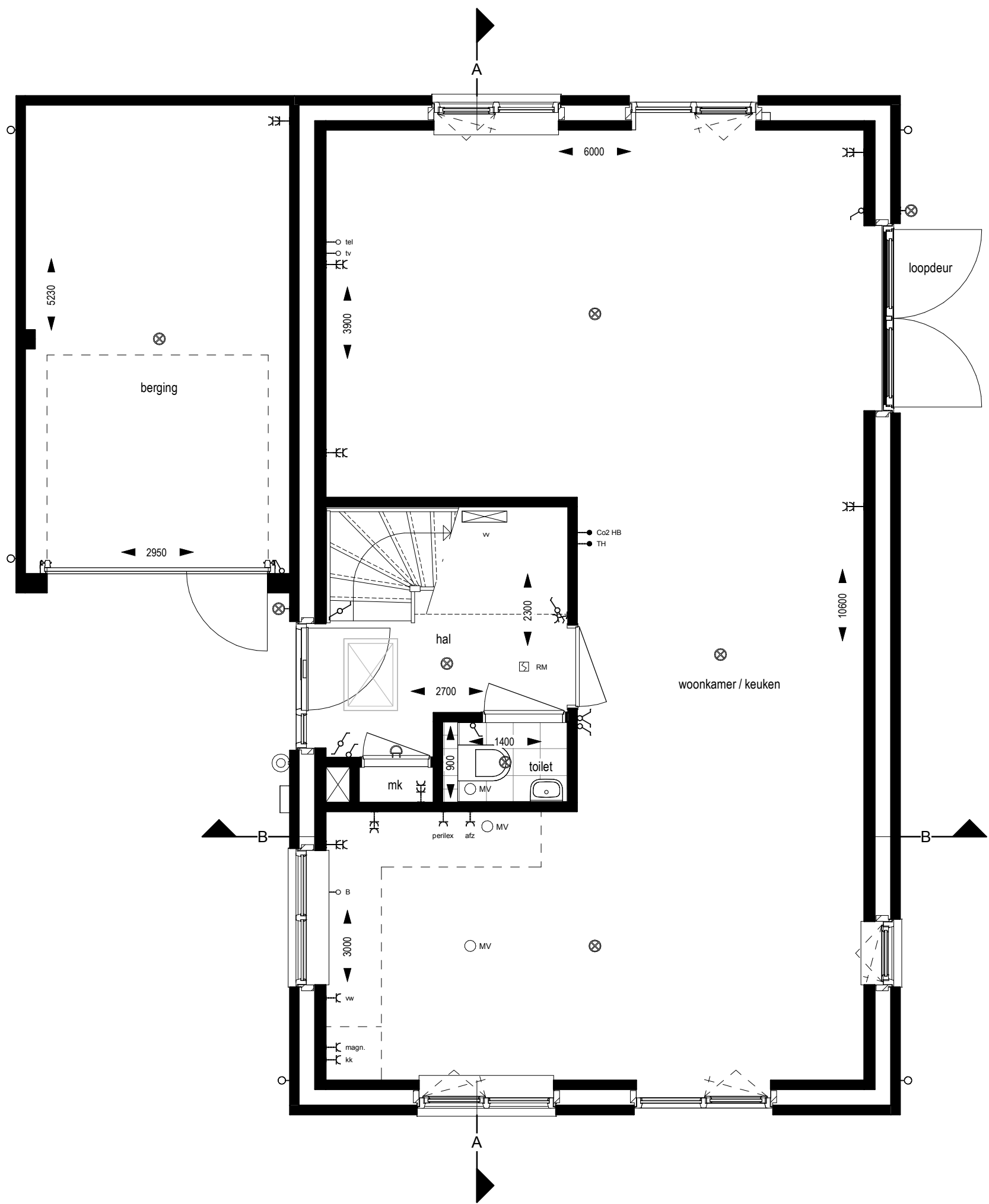
Begane grond
