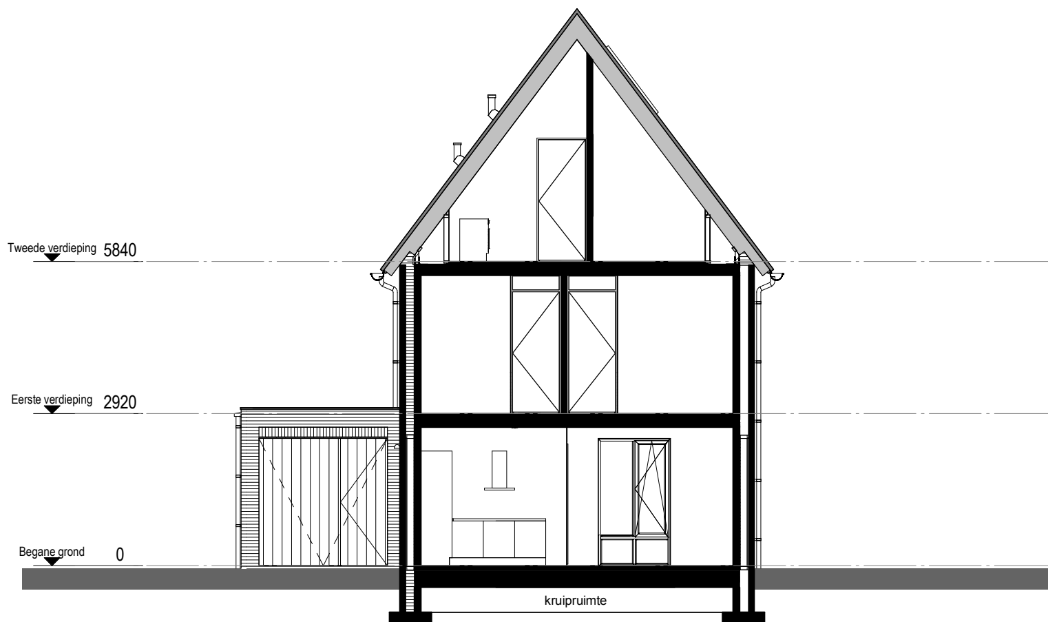
Doorsnede A
